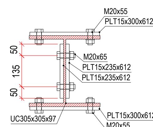
UC305x305x97 BASE PLATE Scale: 1:10
