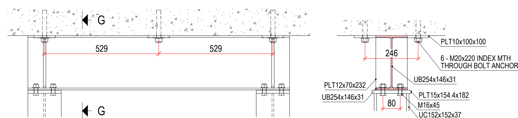
G - G
