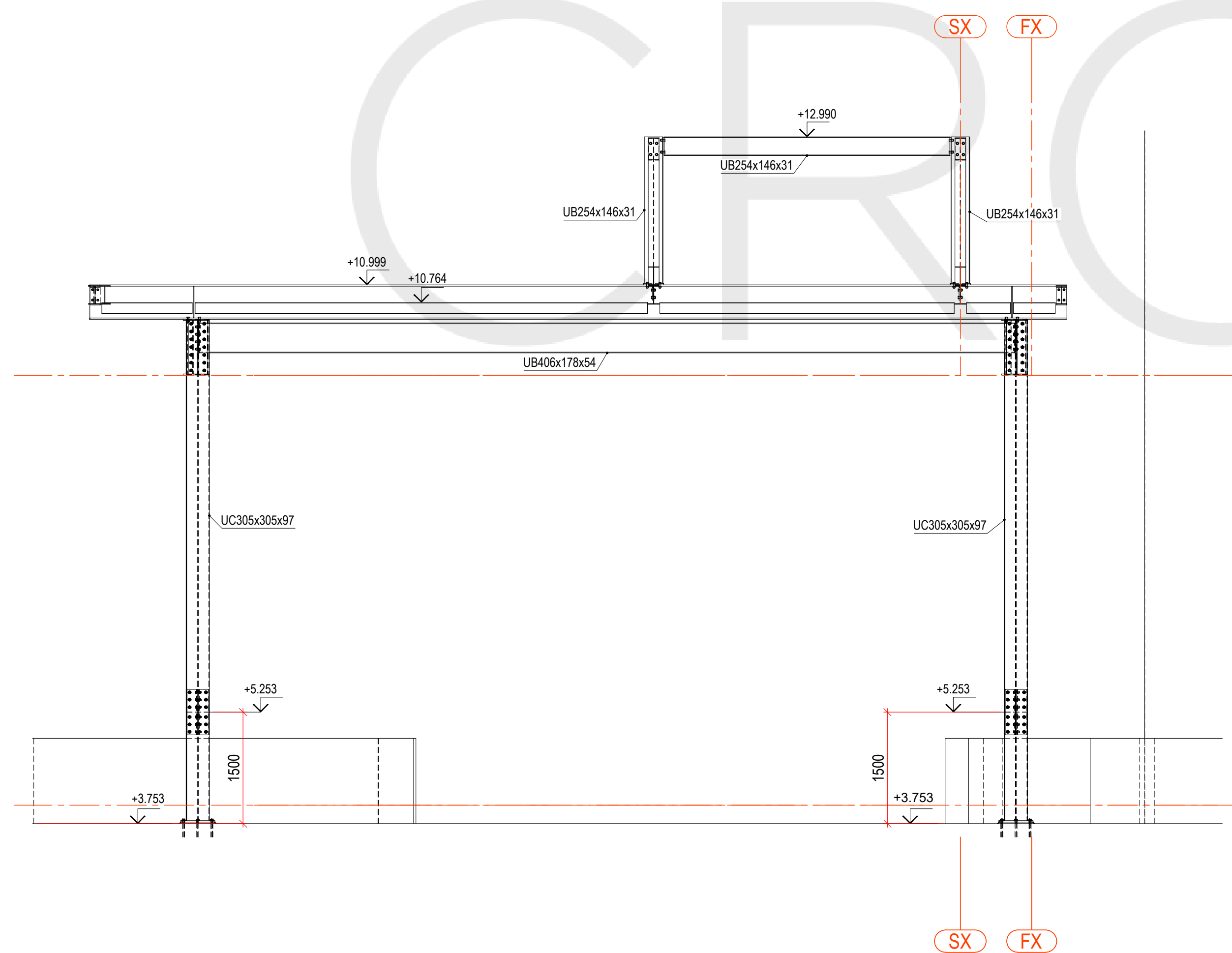
SECTION C-C Scale: 1:50
