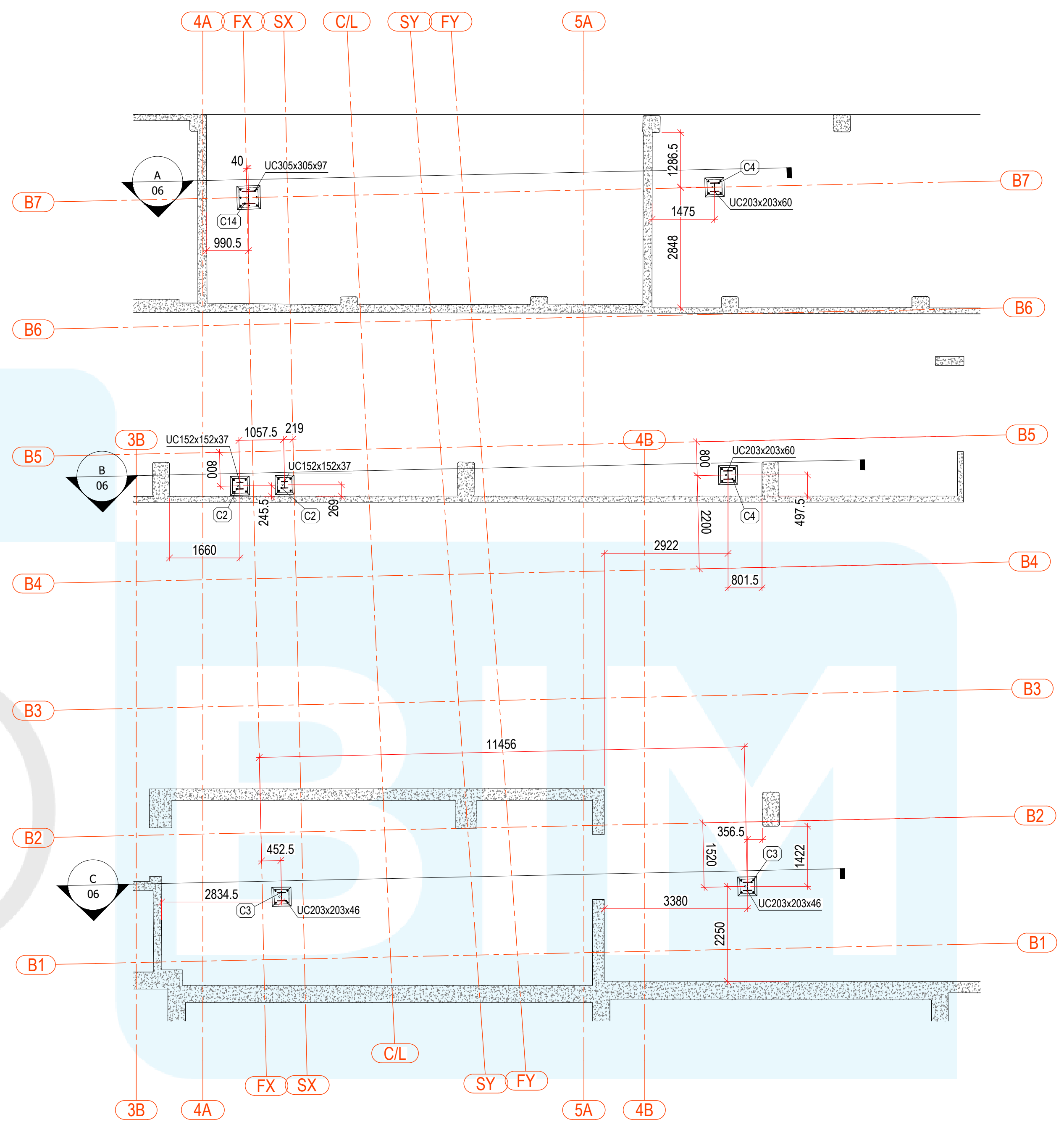
LEVEL B1 Scale: 1:75
