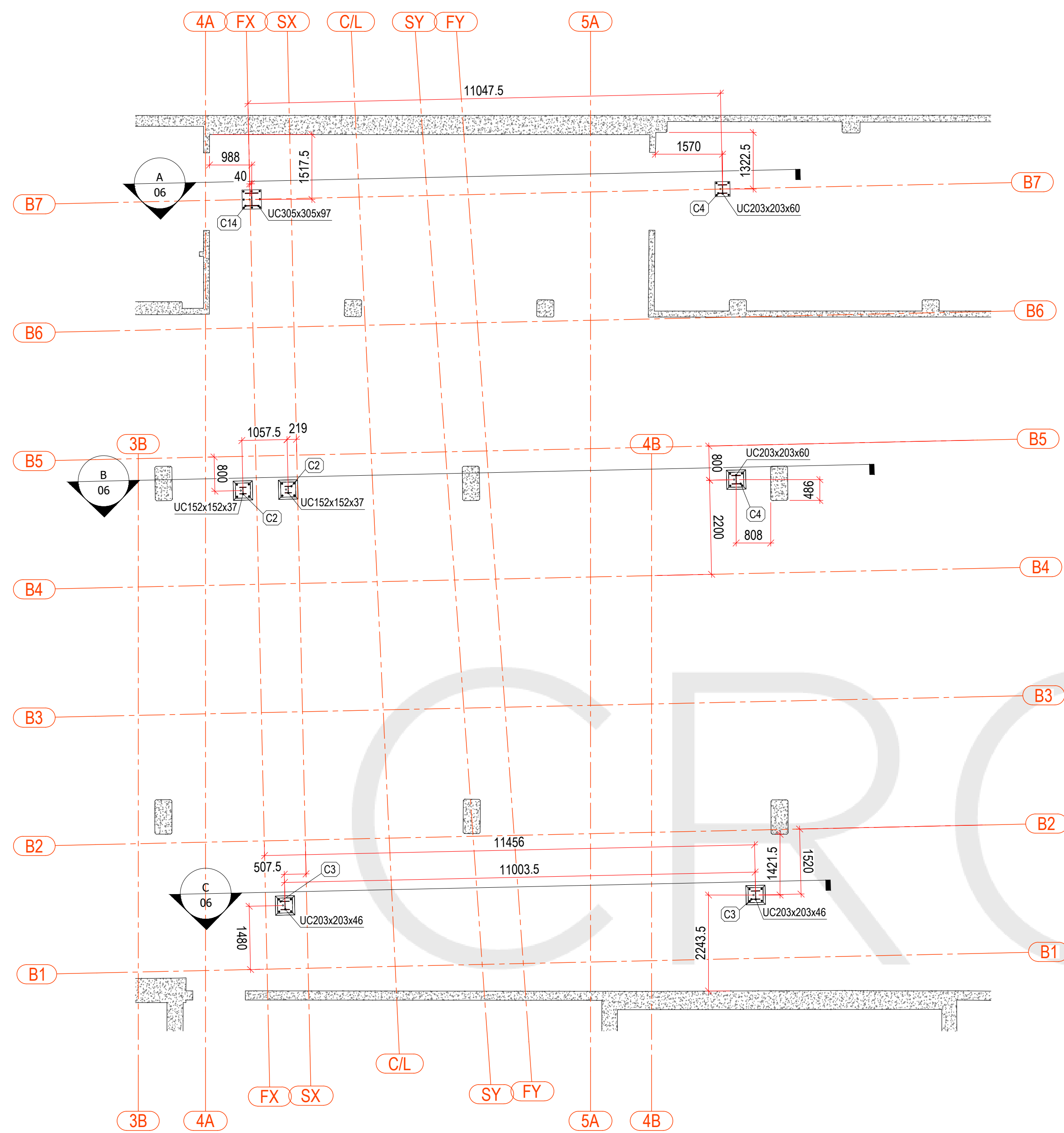
LEVEL B2 Scale: 1:75
