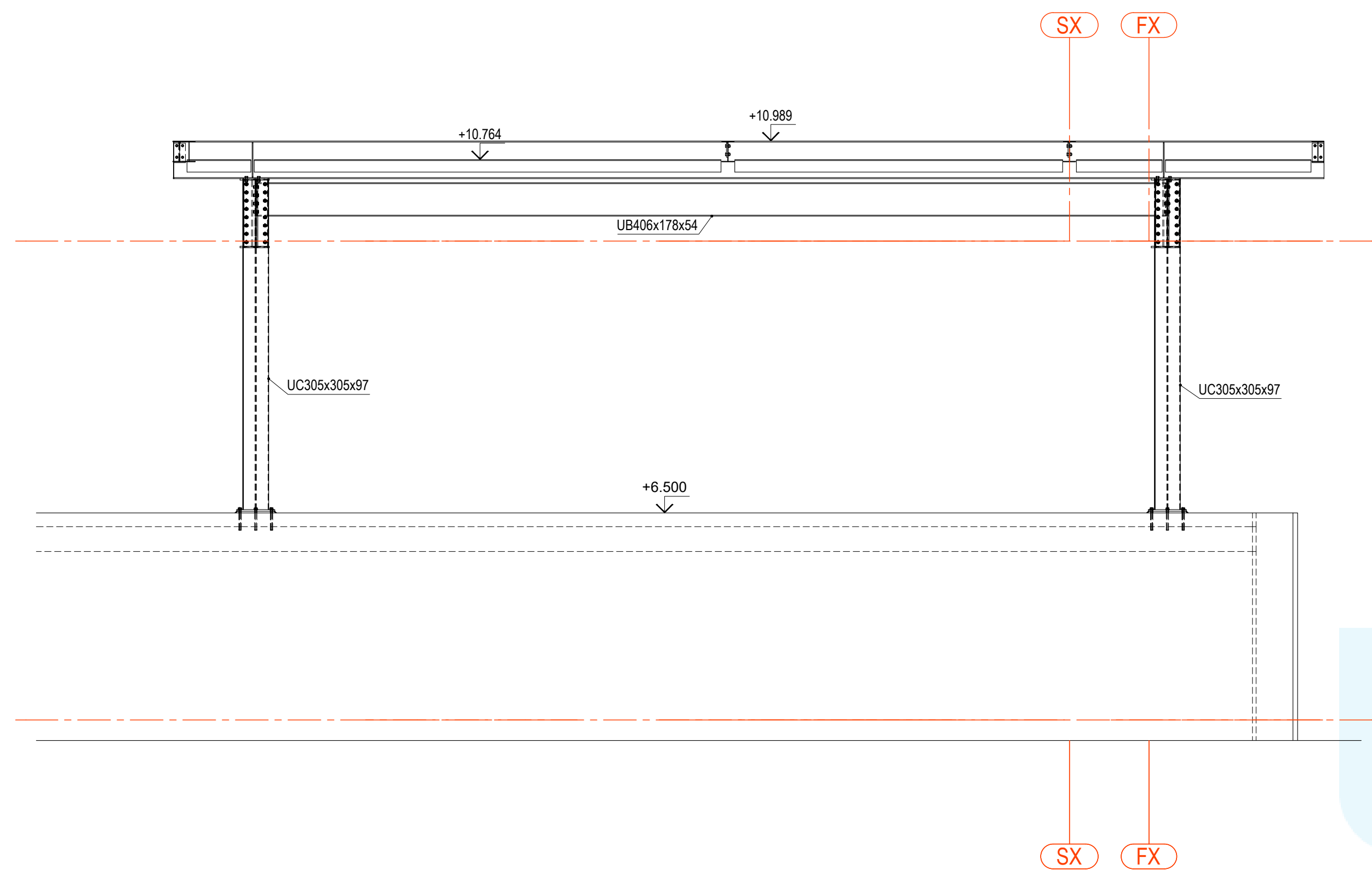
SECTION A-A Scale: 1:50
