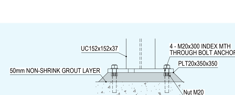
SECTION B-B Scale: 1:50
