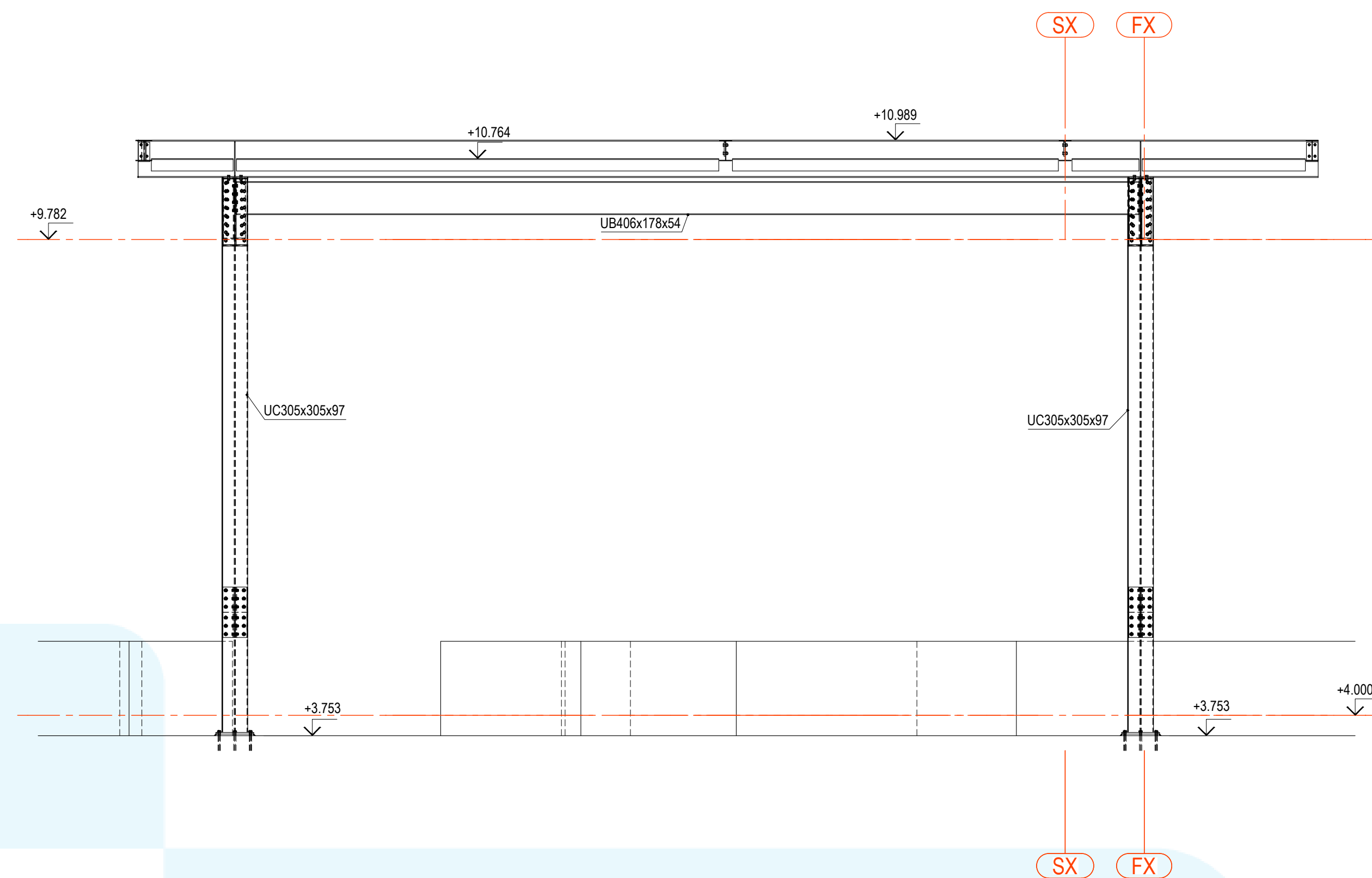
SECTION B-B Scale: 1:50
