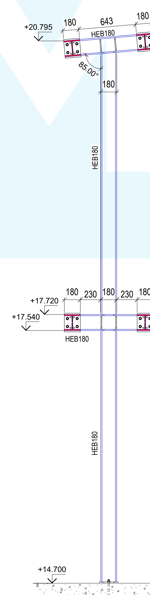
COLUMN TYP 6 Scale: 1:25
