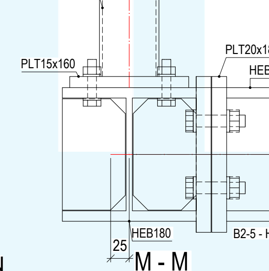
D6 Scale: 1:5
