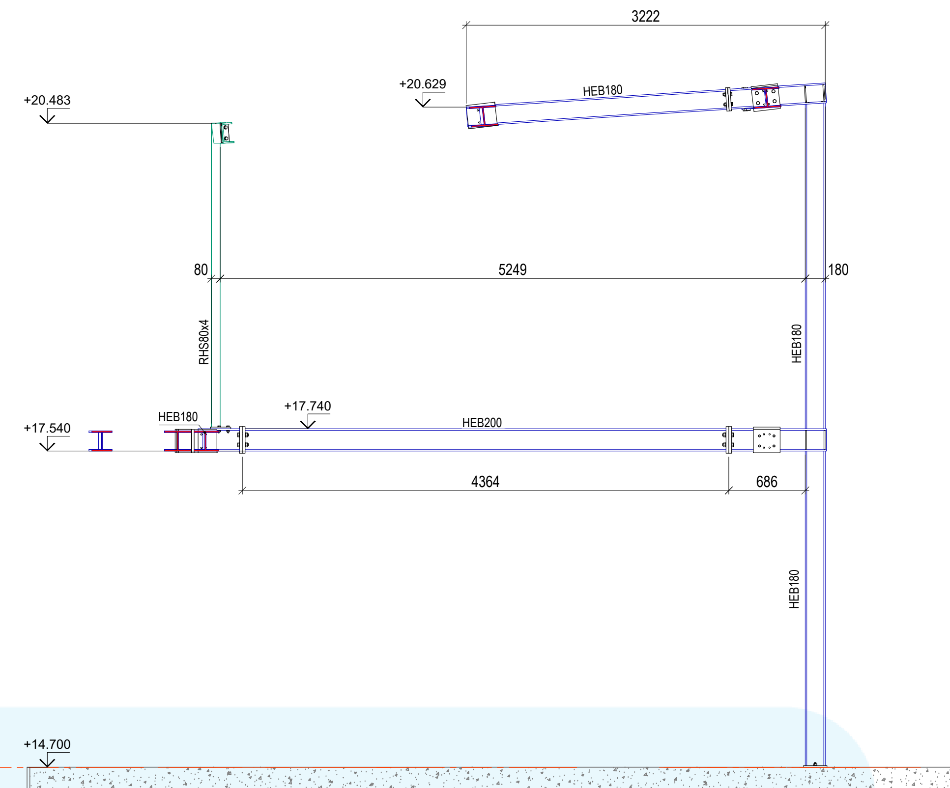
SECTION A-A Scale: 1:33 1/3
