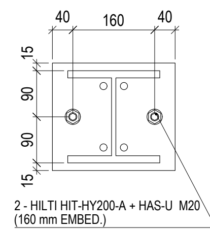
BASE PLATE TYP 1 Scale: 1:7.5
