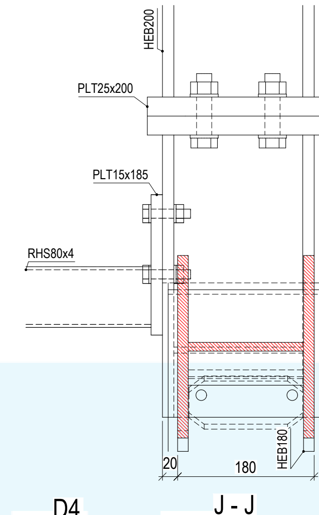
D4 Scale: 1:5
