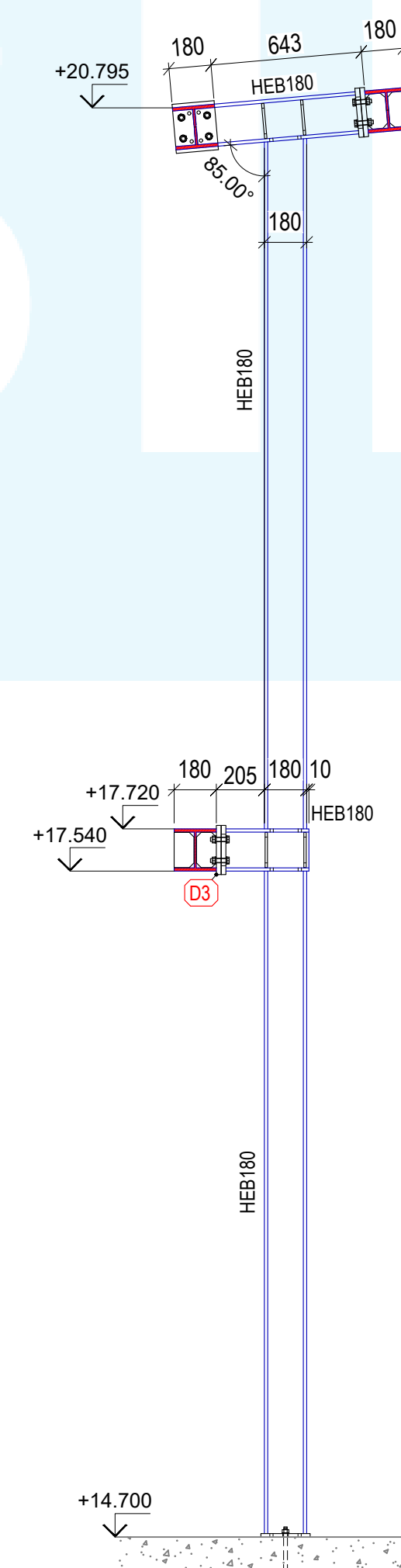
COLUMN TYP 5 Scale: 1:25
