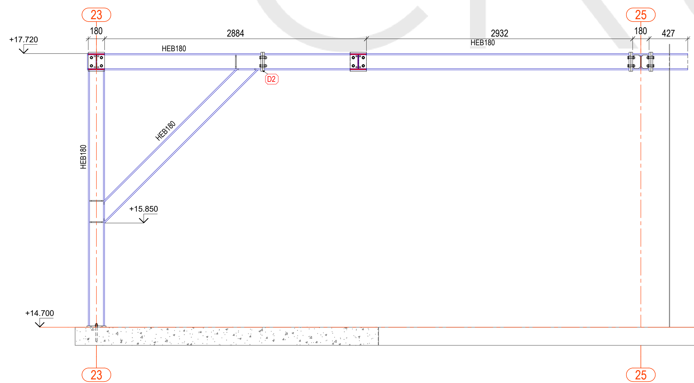
GRID LINE R Scale: 1:25
