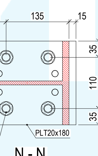
N - N
