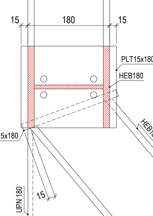
D8 Scale: 1:5
