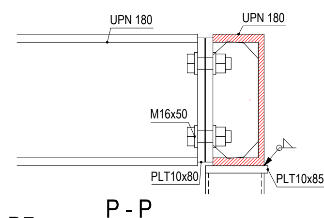
D7 Scale: 1:5
