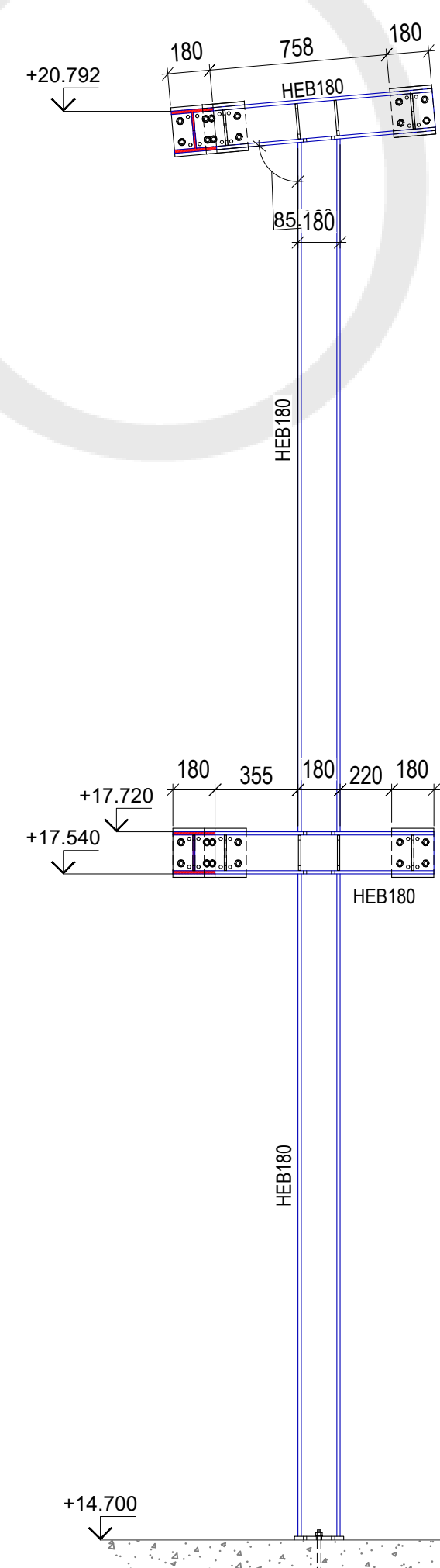
COLUMN TYP3 Scale: 1:25
